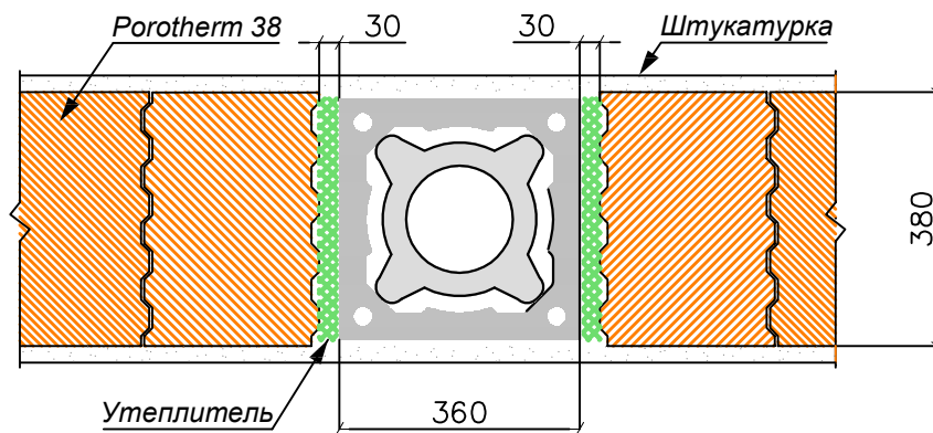
Перевязка стены из Porotherm 38 с ДЫМОХОДНОЙ СИСТЕМОЙ Schiedel ISOTOR 16L
